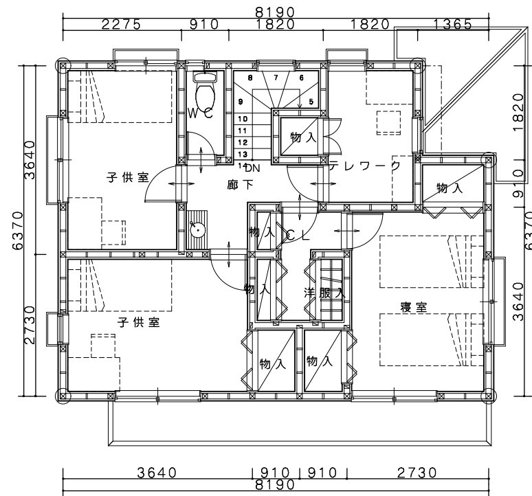
2階平面図
