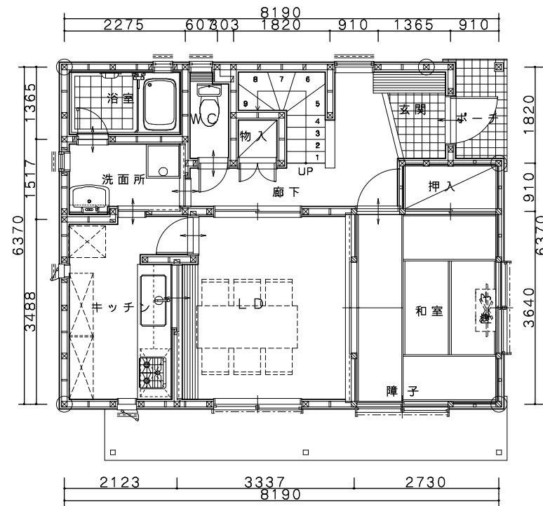
1階平面図
