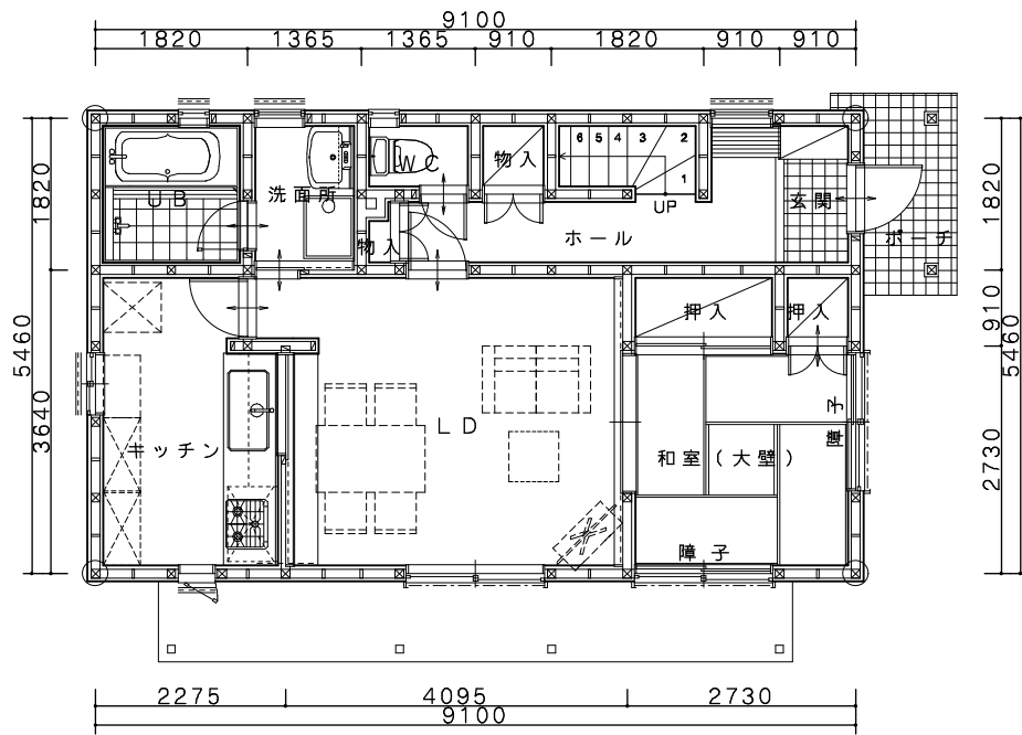
1階平面図
