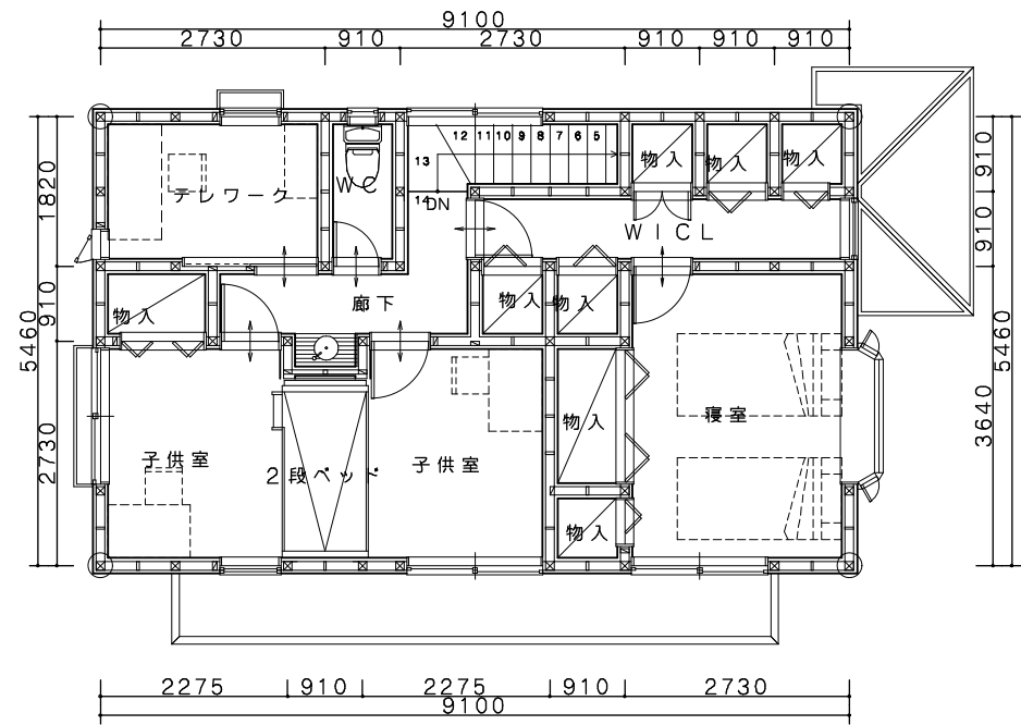
2階平面図
