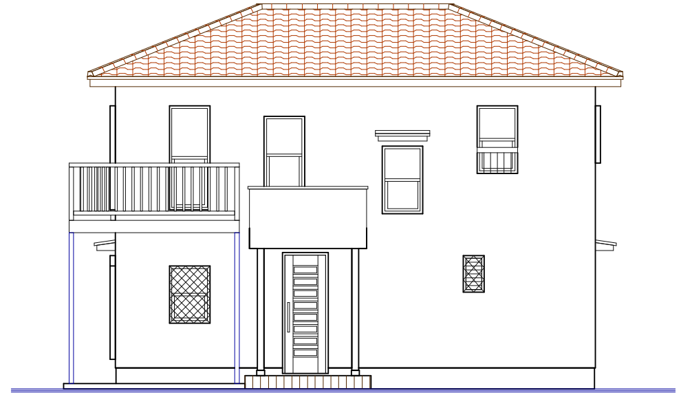
東側立面図
