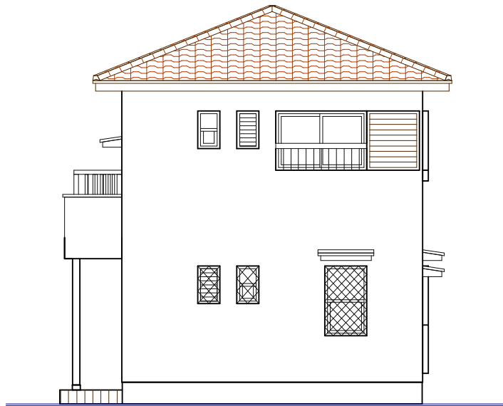
北側立面図
