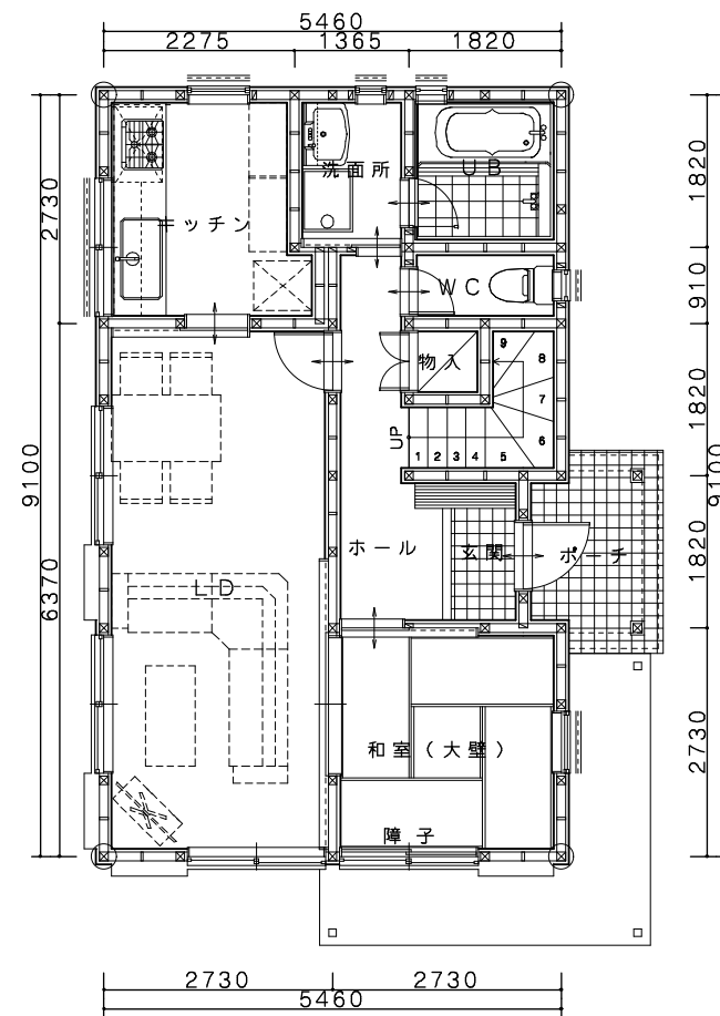
1階平面図
