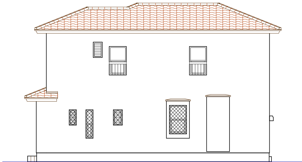
北侧立面图
