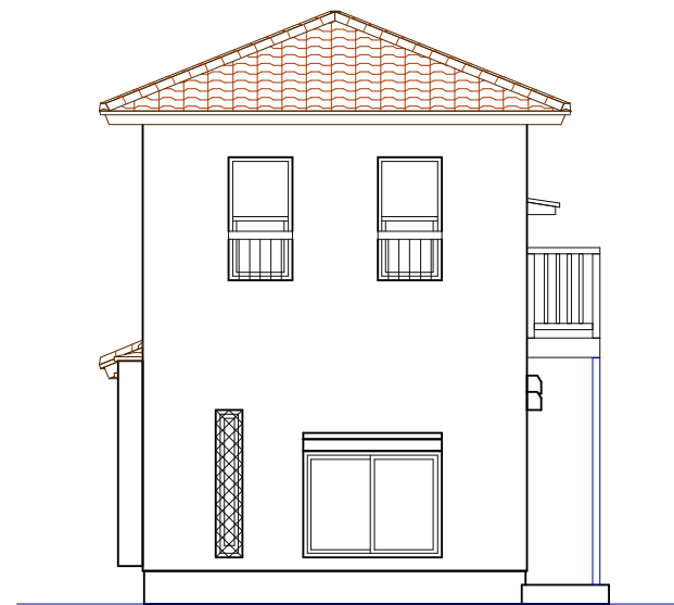
西侧立面图
