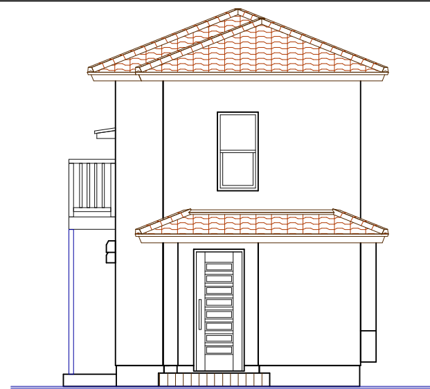
东侧立面图
