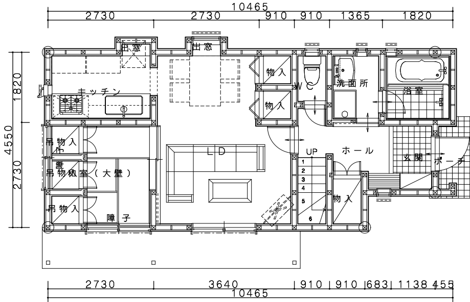
1階平面図
