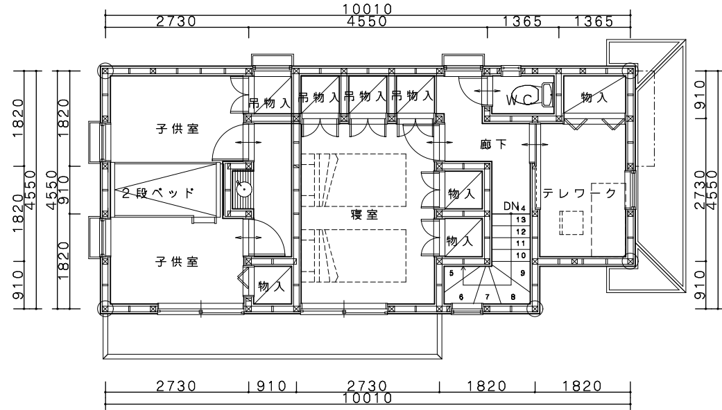
2階平面図
