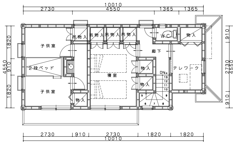
2階平面図
