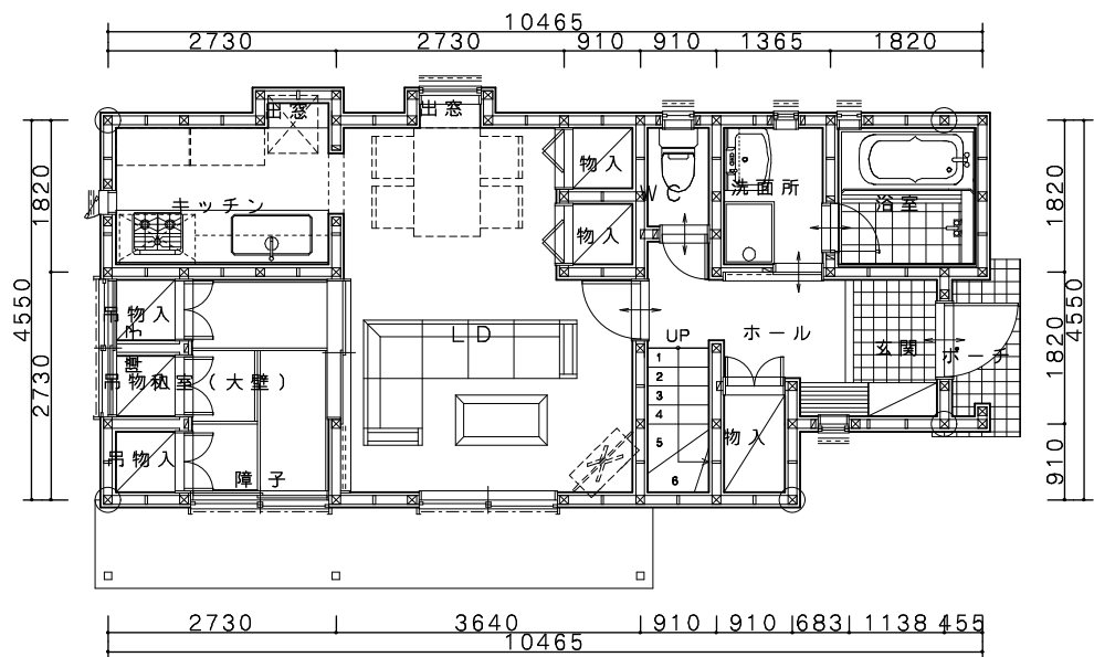
1階平面図
