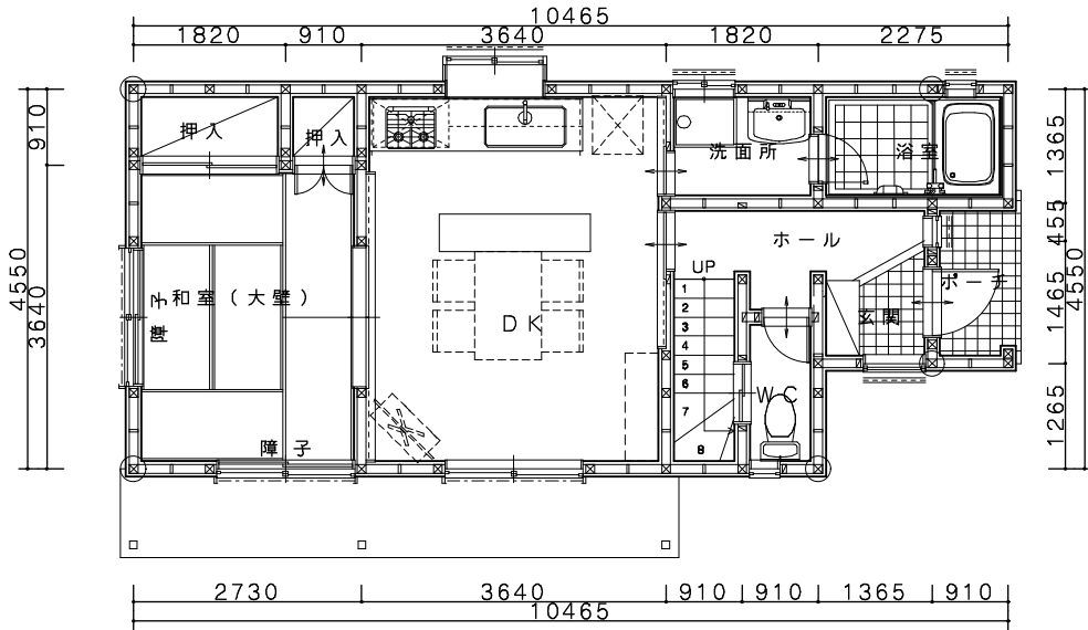
1階平面図
