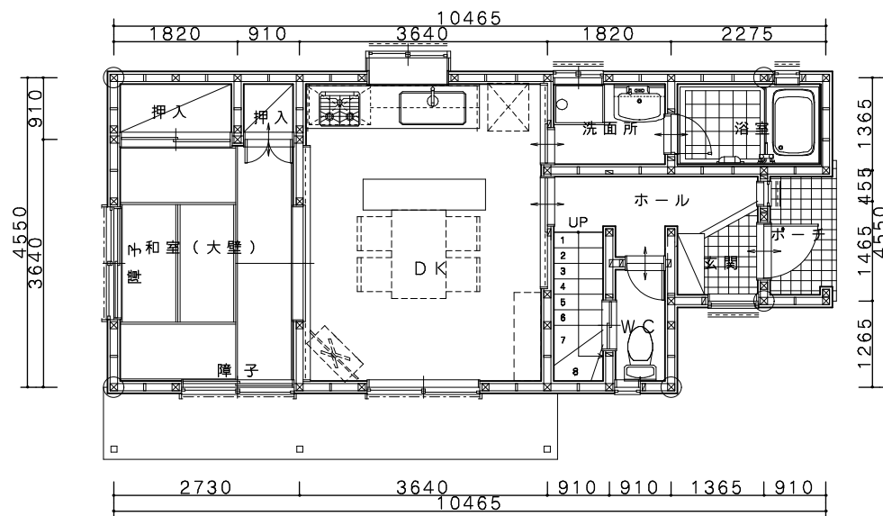
1階平面図
