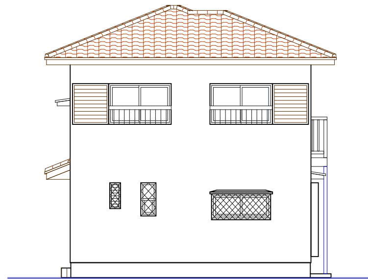
西側立面図
