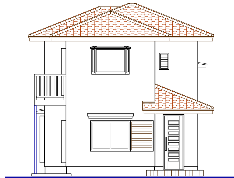
東側立面図
