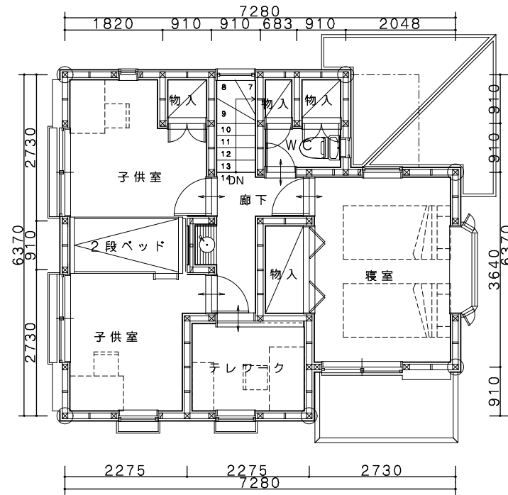
2階平面図
