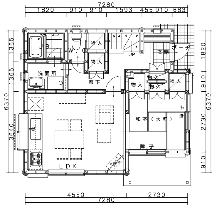
1階平面図
