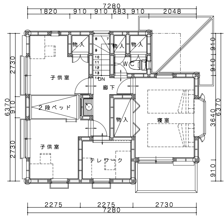
2階平面図
